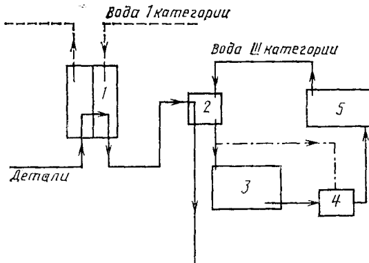
Схема финишной промывки (подача воды и перемещение деталей)
